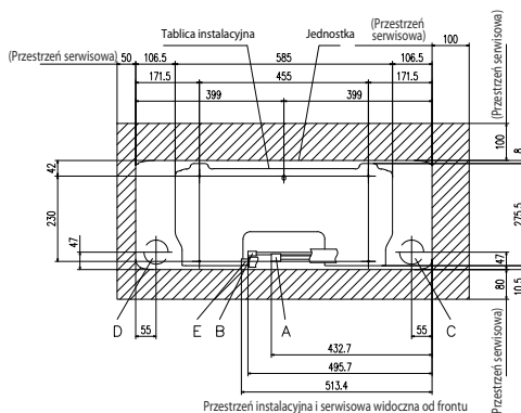
Przerzeń instalacyjna i serwisowa widoczna od frontu
